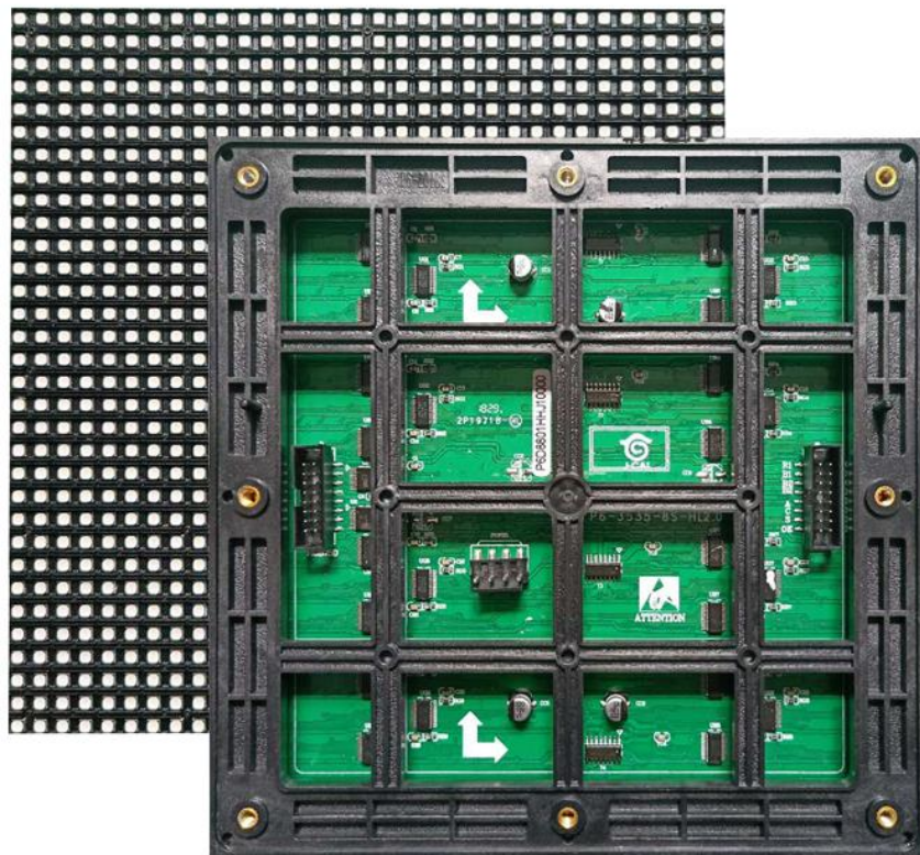
P6-192*192mm-3535
